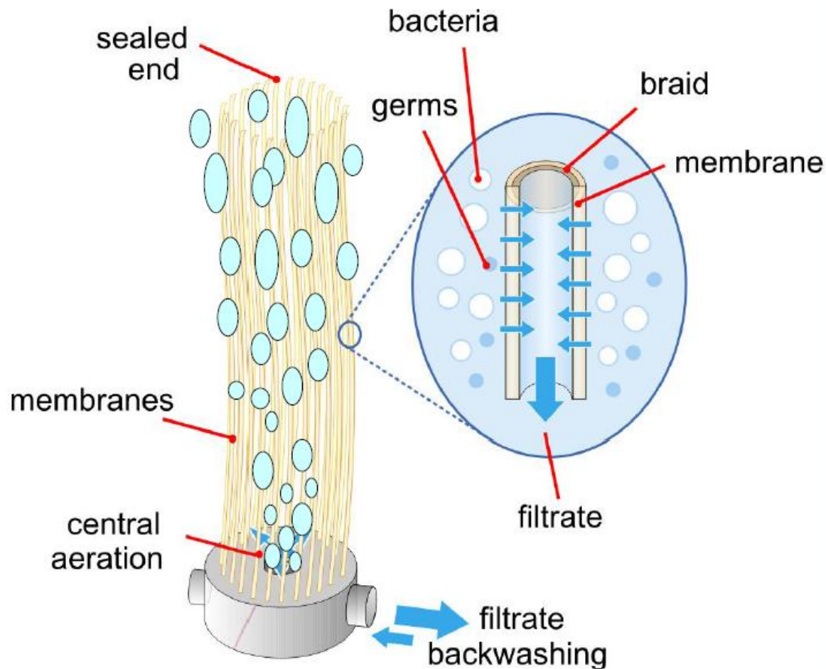
Membrane bundle
