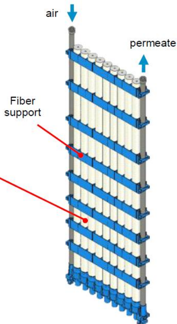
Module row
